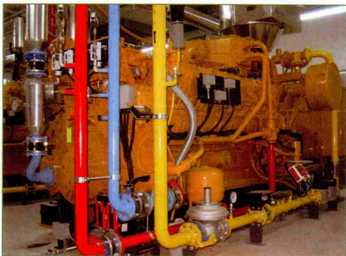
Impianto di cogenerazione
